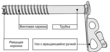
Рис. 2. Идентификация изделия
