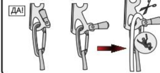
Рис. 11. Проверка изделия
