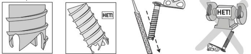
Рис. 12. Заточка коронки
