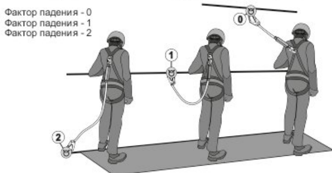
Рис. 13. Графическая схема к определению фактора падения
