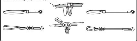
Рис. 10. Регулировка длины
